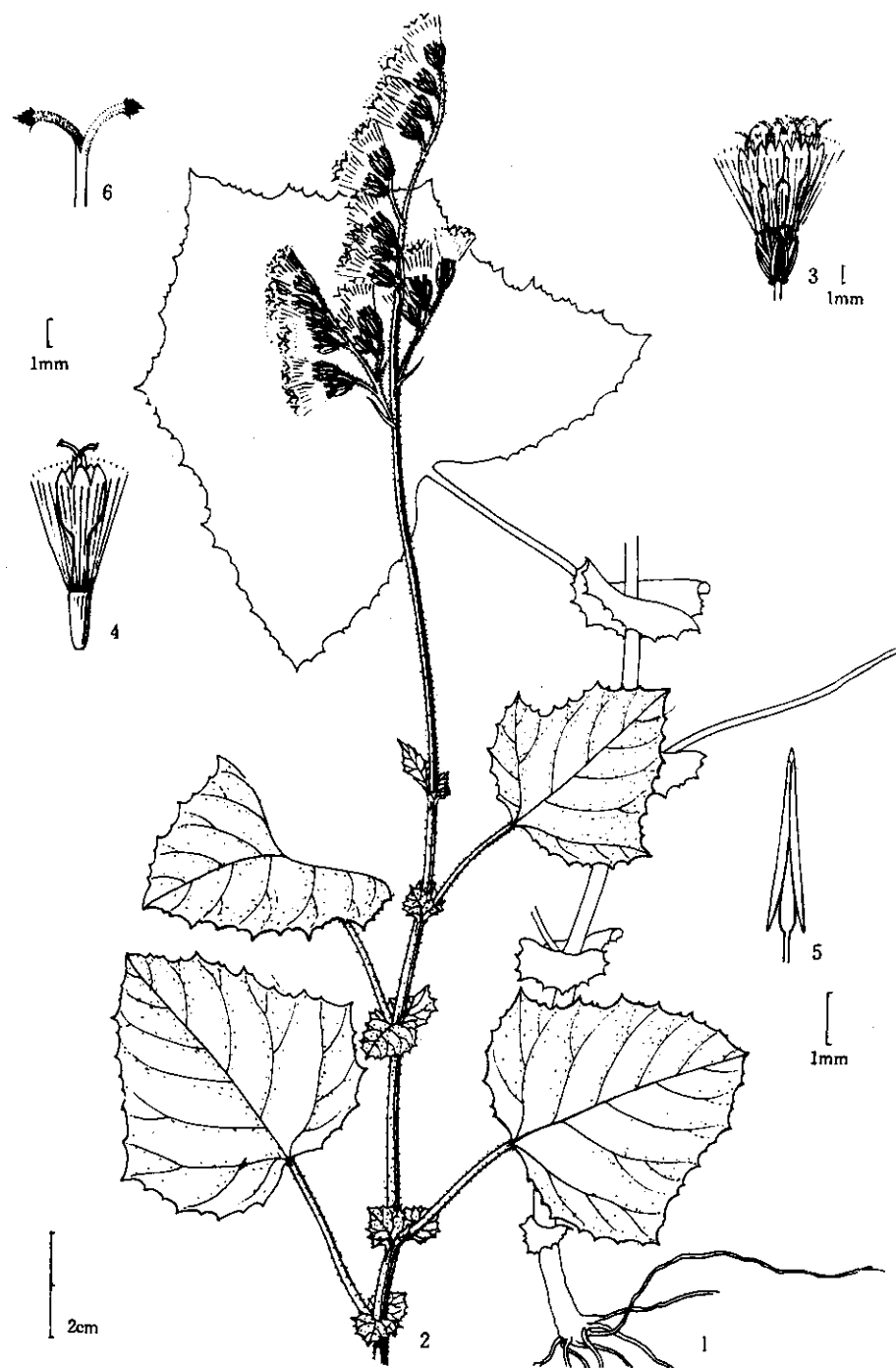
图4 耳柄尾药菊 1, 2. 植株; 3. 头状花序; 4. 管状花; 5. 花药; 6. 花柱分枝。(张泰利绘) Fig. 4 Synotis otophylla 1, 2. habit; 3. capitulum; 4. disc-floret; 5. anther; 6. style-arms.
