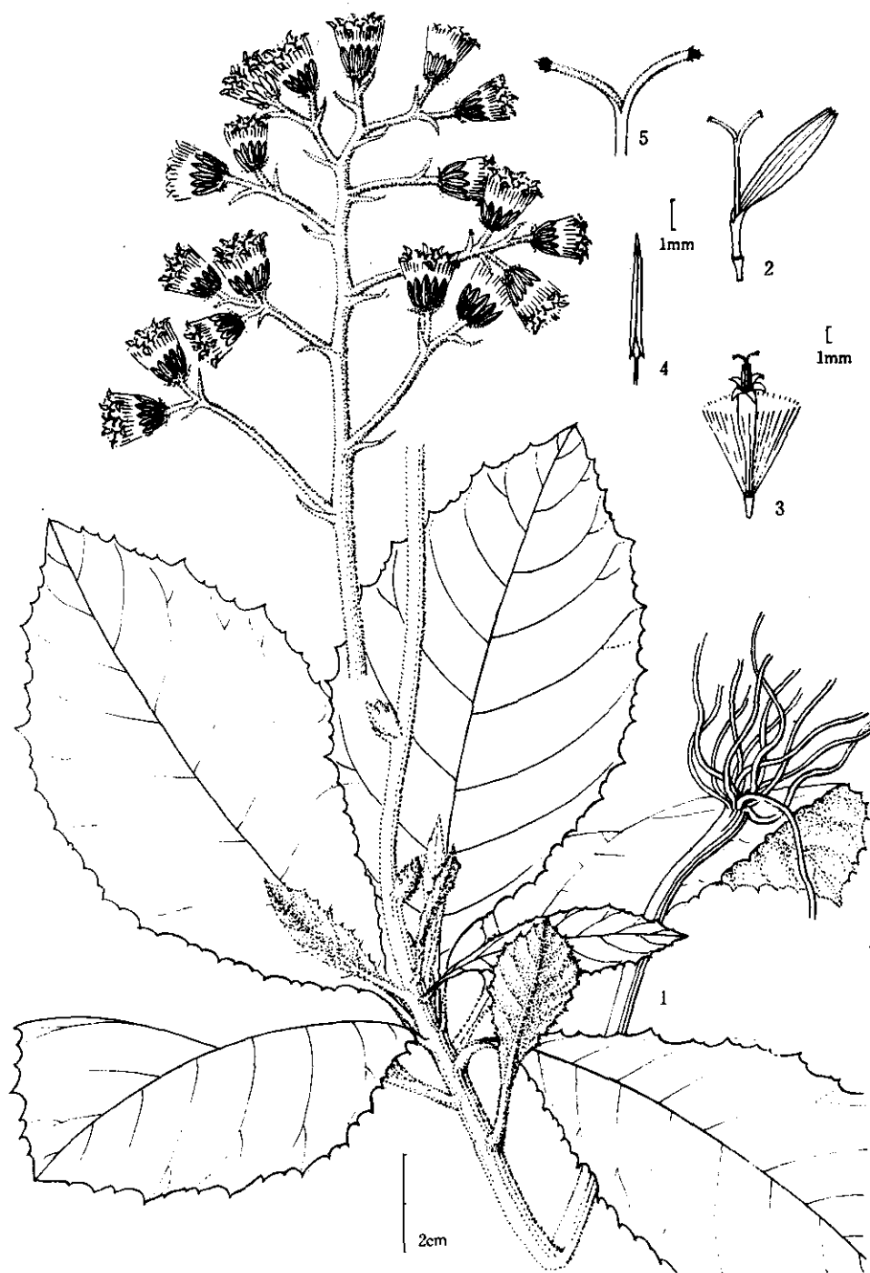
图2 簪毒尾药菊 1. 植株; 2. 舌状花; 3. 管状花; 4. 花药; 5. 花柱分枝。(张泰利绘) Fig. 2 Synotis changiana 1. habit; 2. ray-floret; 3. disc-floret; 4. anther; 5. style-arms.
